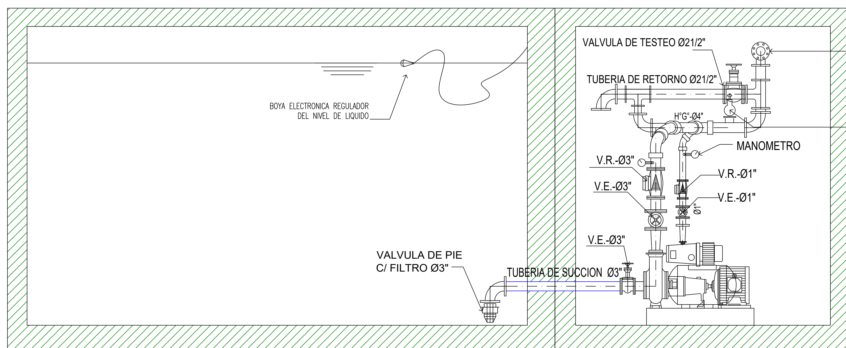
DETALLE CORTE LONGITUDINAL ESC 1/20
