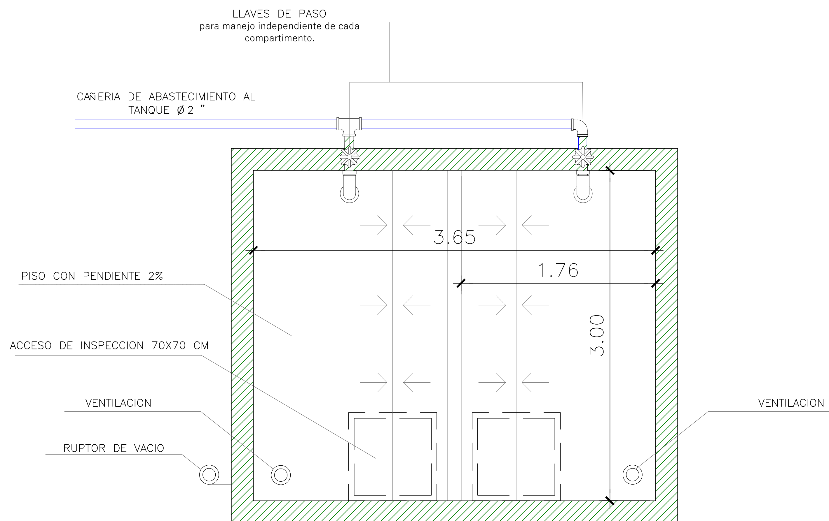
DETALLE TANQUE SUPERIOR ESC 1/20
