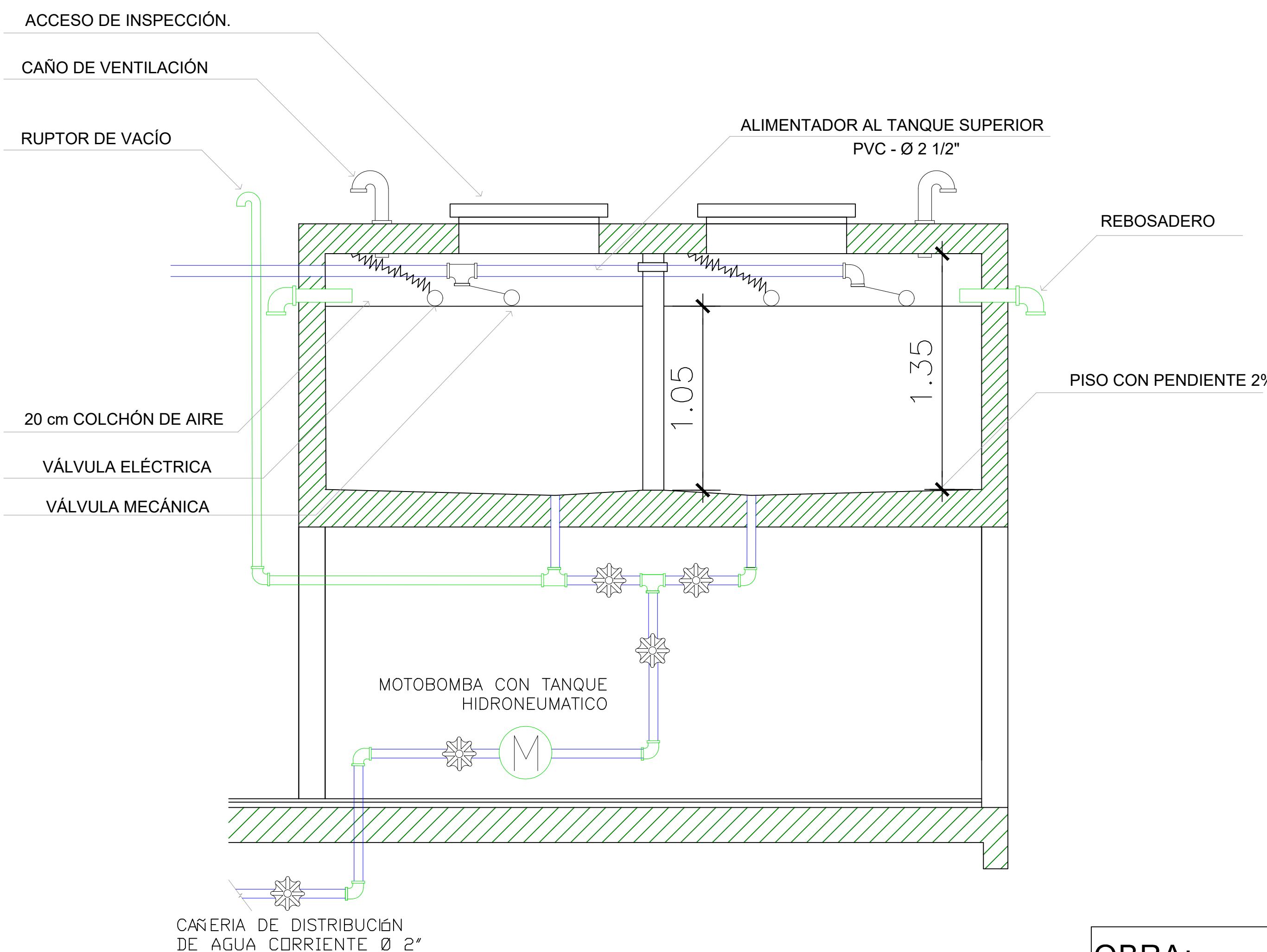
DETALLE CORTE TANQUE SUPERIOR ESC 1/20
